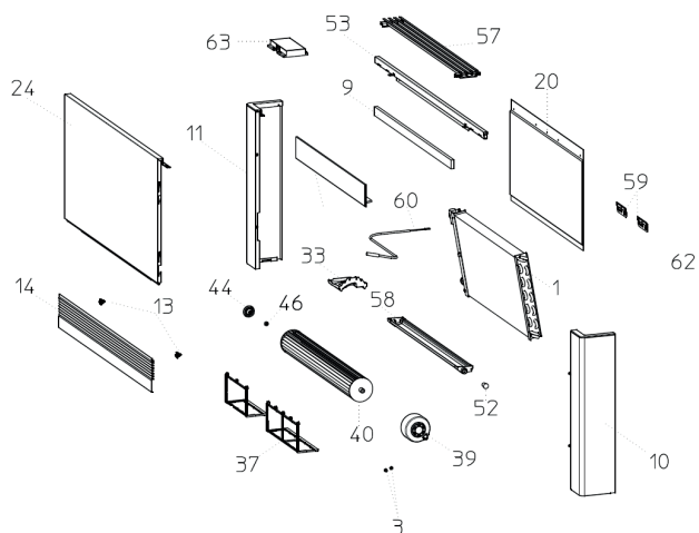
Vayu S 200, 400, 600, 800
