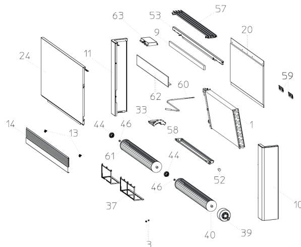
Vayu S 1000
